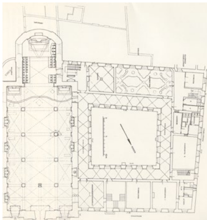
Grundrissplan EG, vor dem Umbau 2003
